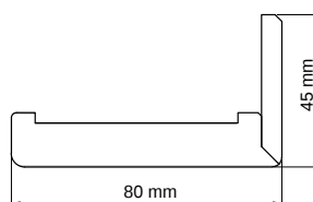
Bară unghiulară pentru tocuri de ușă reglabile - lățime 80 mm
