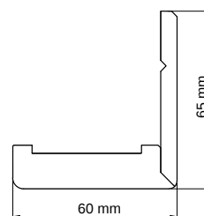
Bară unghiulară de lărgire pentru tocul reglabil - lățime 60 mm
