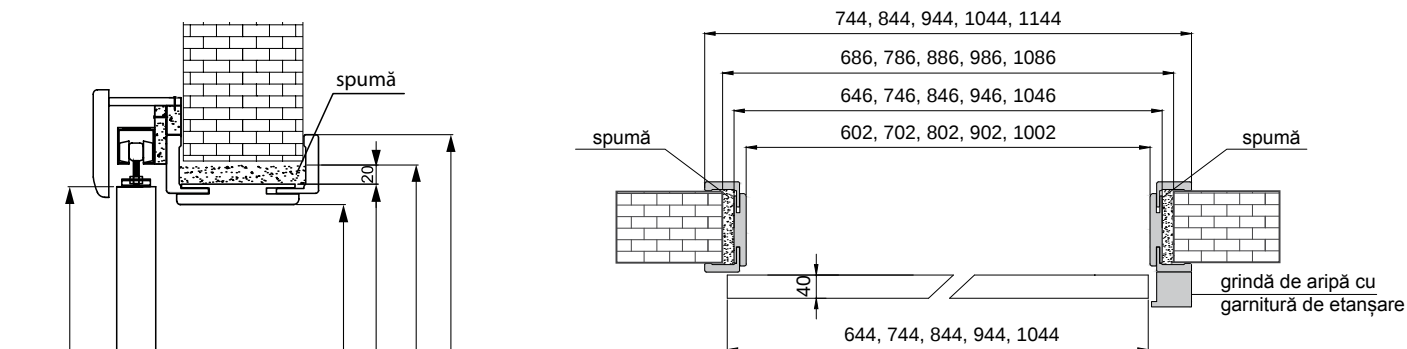
BARĂ DE PROTECȚIE
