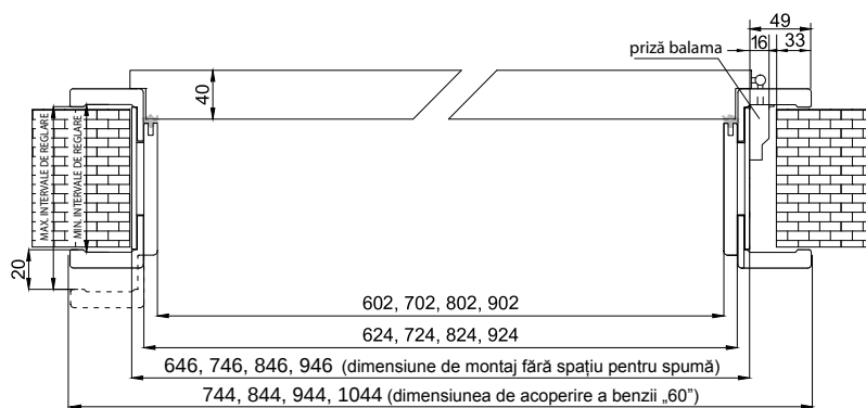
Bară unghiulară pentru tocuri de ușă reglabile - lățime 80 mm
