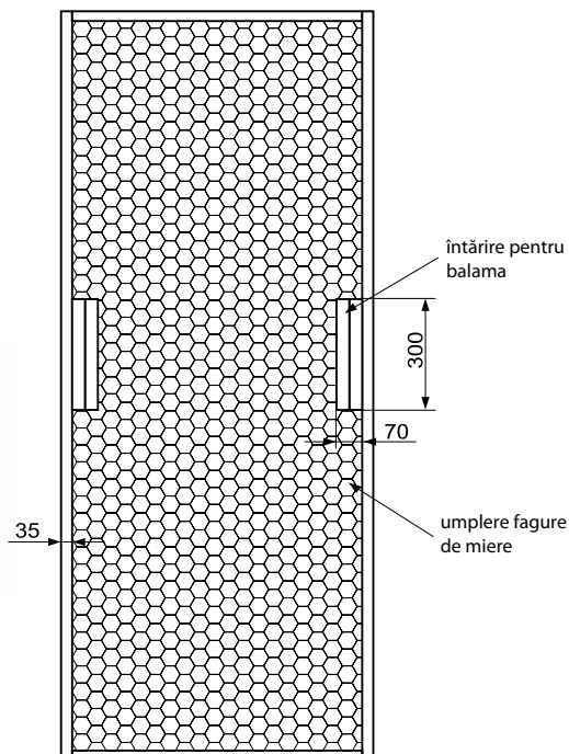
Armătură – placă completă – opțiune pentru costuri suplimentare:
