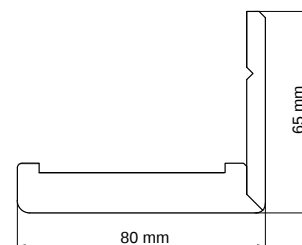
Bară unghiulară de lărgire pentru tocul reglabil - lățime 60 mm
