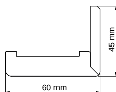
Bară unghiulară pentru tocuri de ușă reglabile - lățime 60 mm
