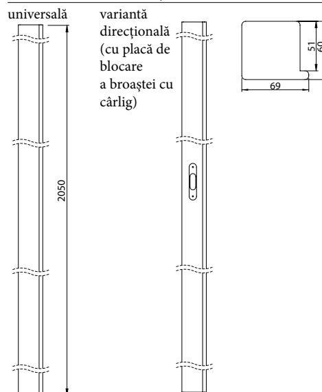
BARĂ DE PROTECȚIE
